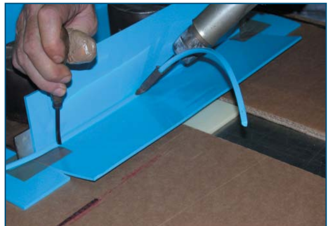
Stabschweißen von Profilen
