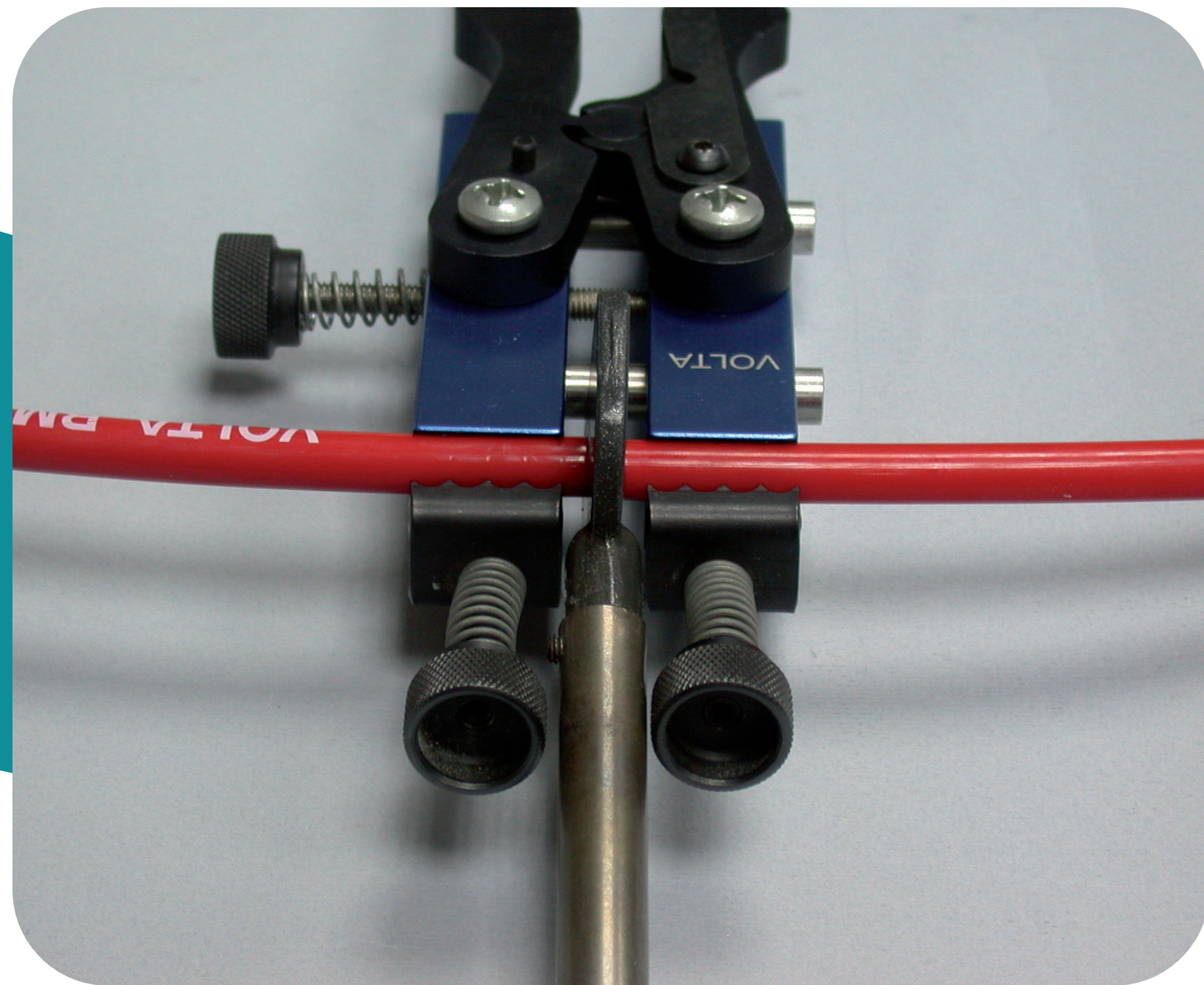
R8 Mini pliers for smaller profiles
