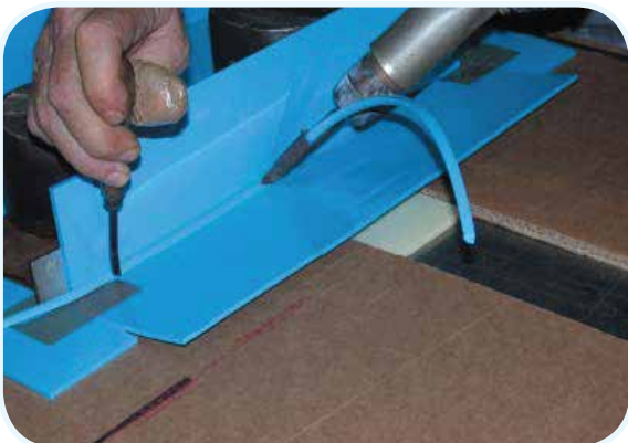
Soudage de tasseaux avec électrode
