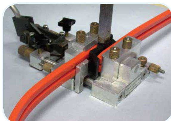
Soudure par recouvrement Easy Overlap
