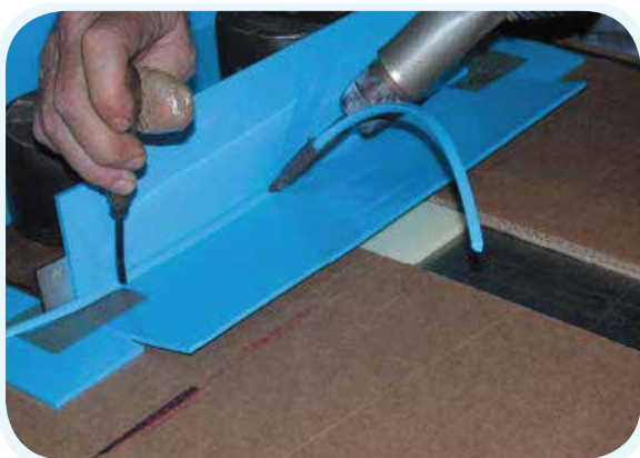
FT-Stabschweißen von Elektrodenschweißgerät Stollen
